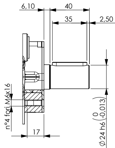
Detailed shaft view Vista dettagliata albero
